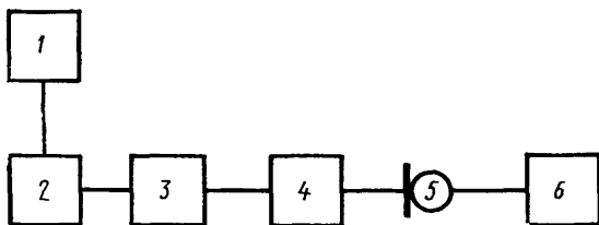
1—частотомер; 2—генератор; 3—магазин затухания; 4—электростатический возбудитель; 5—поверяемый микрофон; 6—электронный вольтметр.
