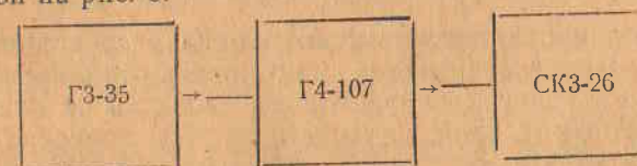
Рис. 8. Структурная схема измерения девиации частоты генератора в режиме внешней частотной модуляции.
