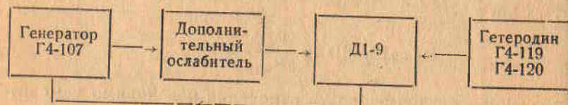
Рис. 5. Структурная схема измерения погрешности установки ослабления аттенюатора.
